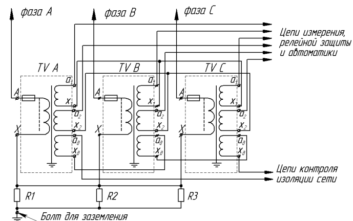
Рисунок А.4 Принципиальная электрическая схема трехфазной группы ЗХЗНОЛП
