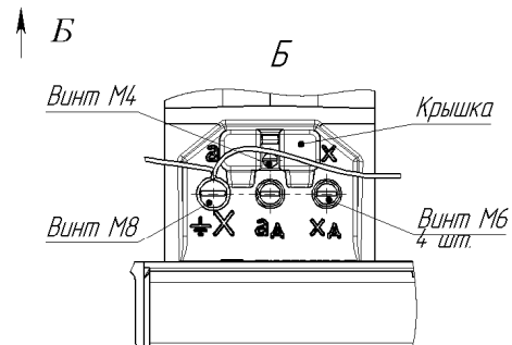
Рисунок А.1 Общий вид трехфазной группы ЗхЗНОЛП
