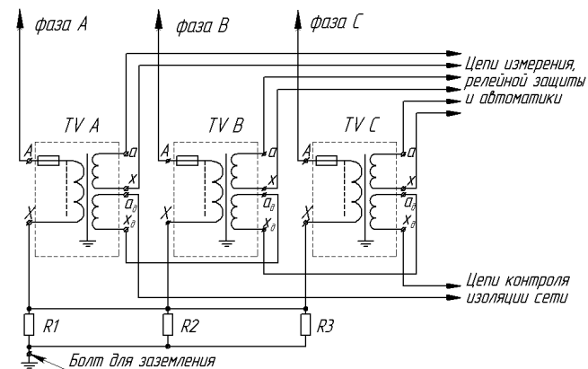
Рисунок А.2 Принципиальная электрическая схема трехфазной группы ЗхЗНОЛП
