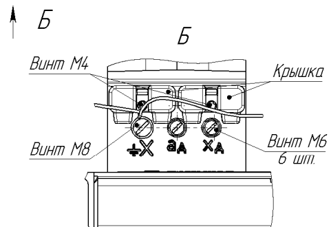
Рисунок А.3 Общий вид трехфазной группы ЗХЗНОЛП
