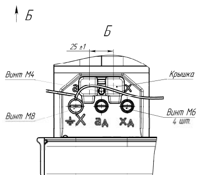
Рисунок А.1 Общий вид трехфазной группы ЗХЗНОЛ.06
