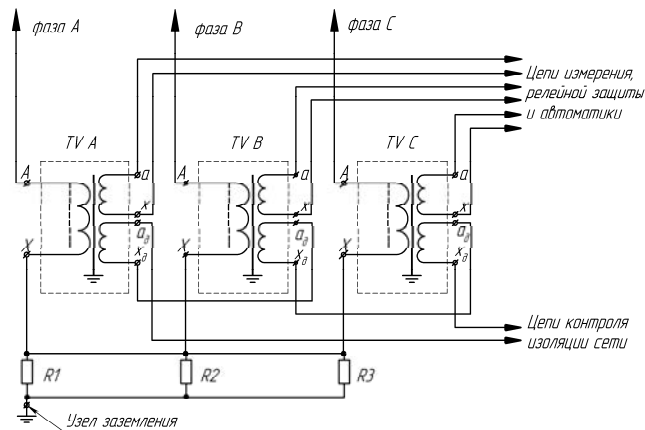
Рисунок А.2 Принципиальная электрическая схема трехфазной группы ЗХЗНОЛ.06
