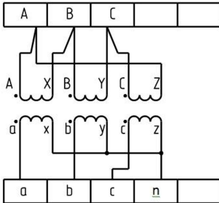
Рисунок 1 – Электрическая схема.
